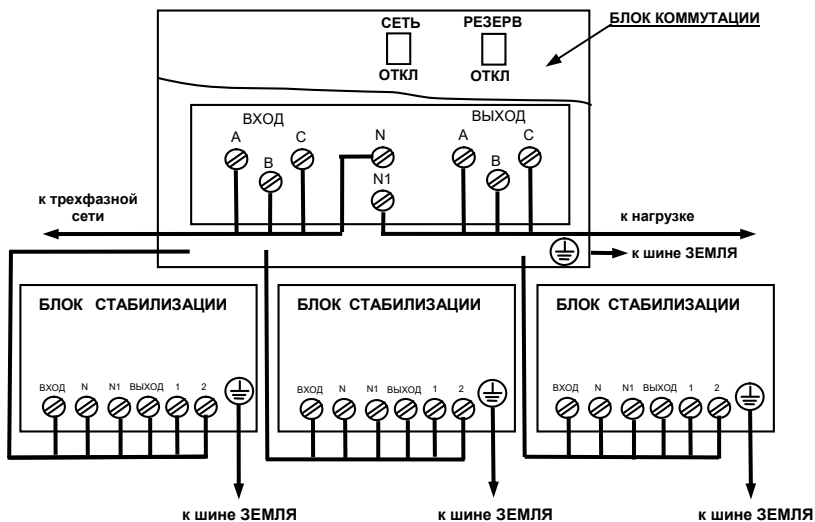
Рисунок 6.1 Схема подключения стабилизатора R13500-3 К (R15000-3 К, R18000-3 К, R22500-3 К, R24000-3 К, R30000-3 К)
