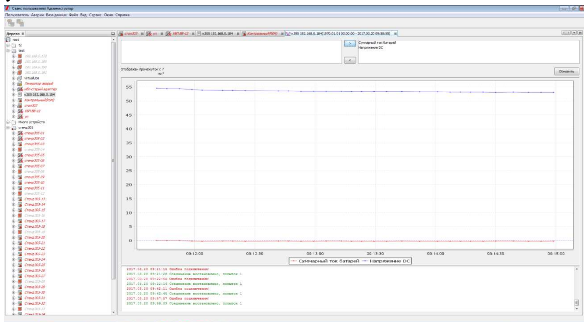
Рисунок 5.22 пример графика параметров АКБ
