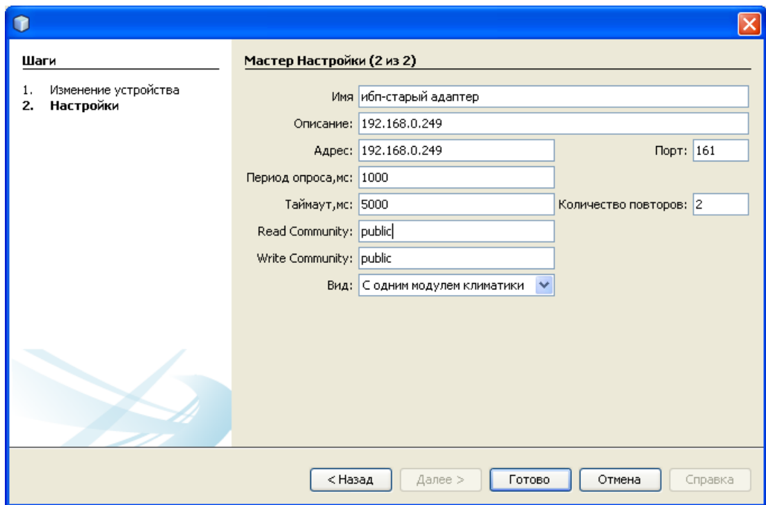
Рисунок 5.4 настройка сетевых параметров ИБП
